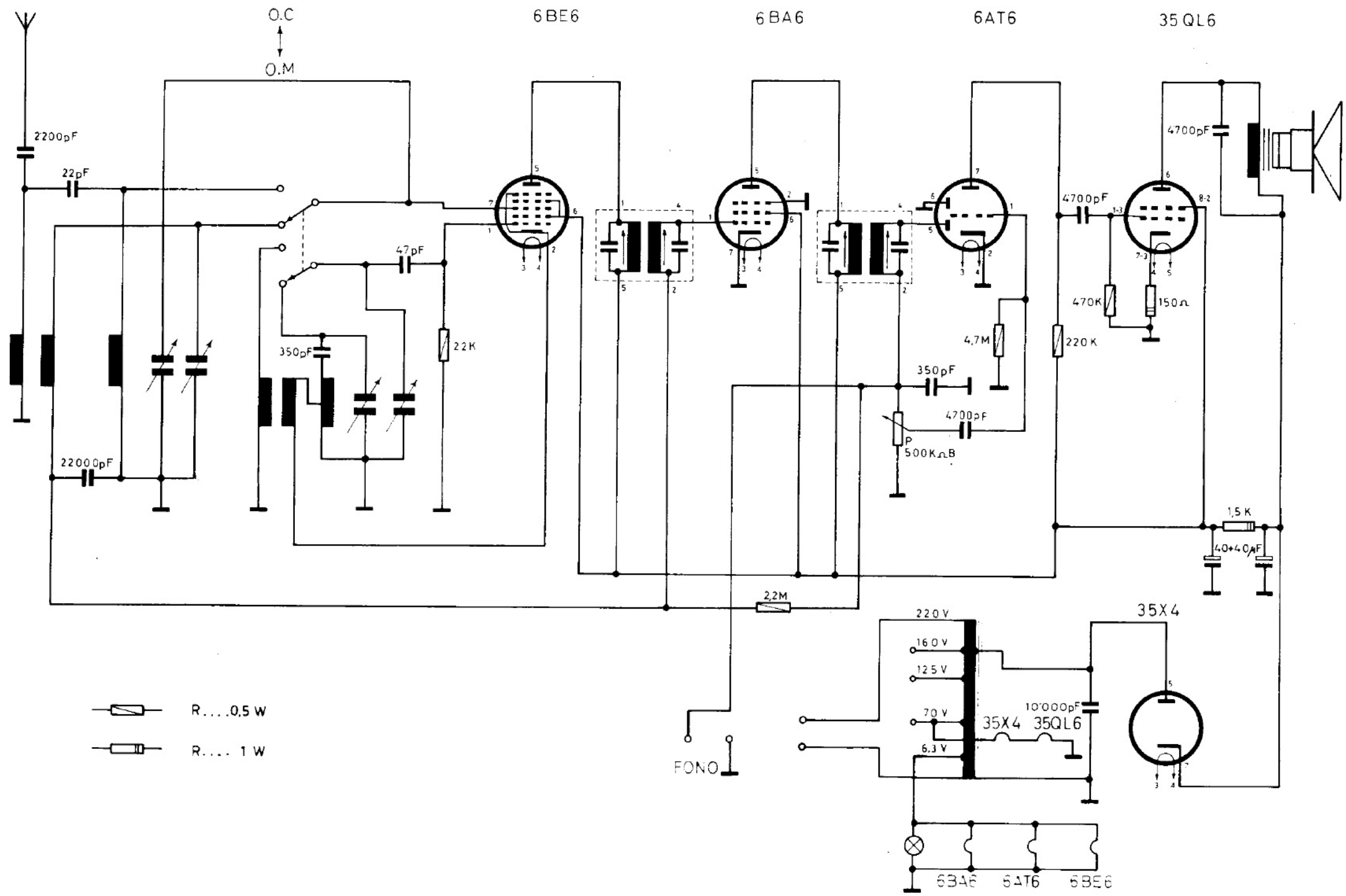
SCHEMA ELETTRICO DEI RADIORICEVITORI G.B.C. AR/1A KITTY e AR/8A WONDERFUL
